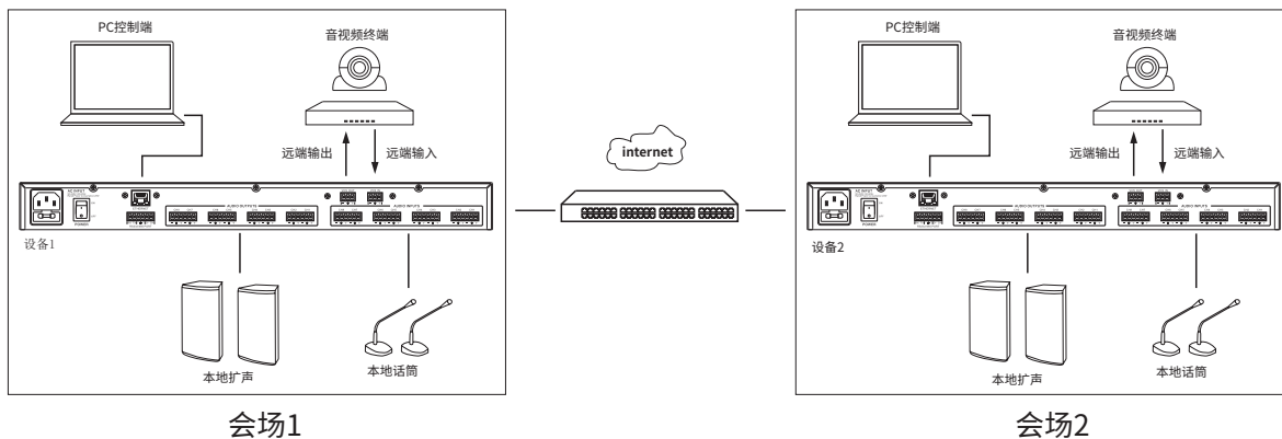
AC回声消除系统连接图
